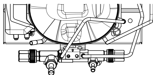
Version avec kit de raccordement
