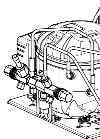
Version avec kit de raccordement et mini pressostat
